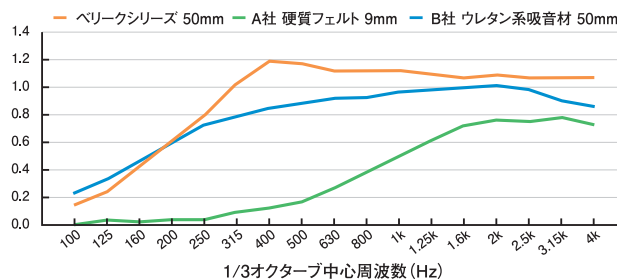
残響室法吸音率データ
